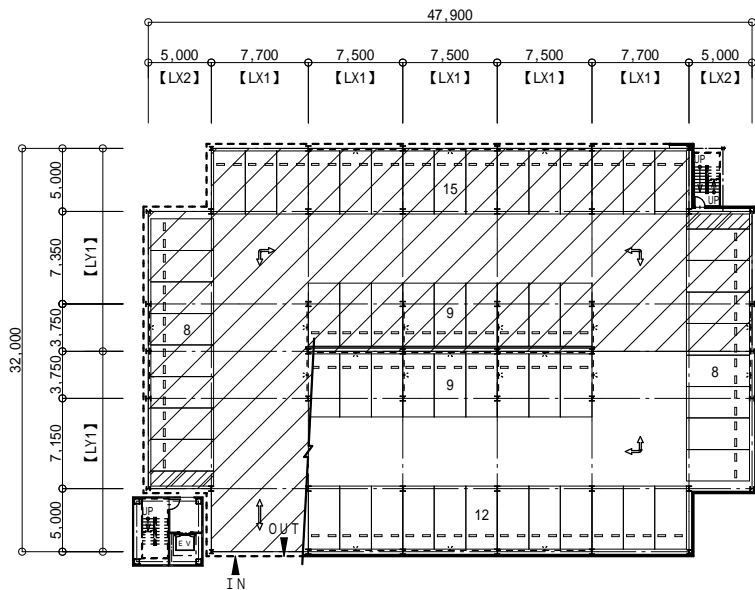
1階 平面図
