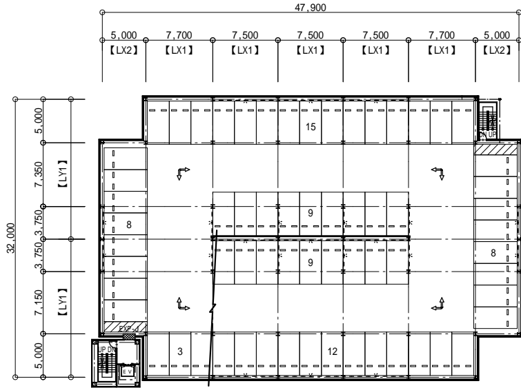
2 ~ 6階 平面図
